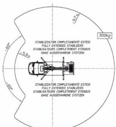
Abstützung beidseitig
